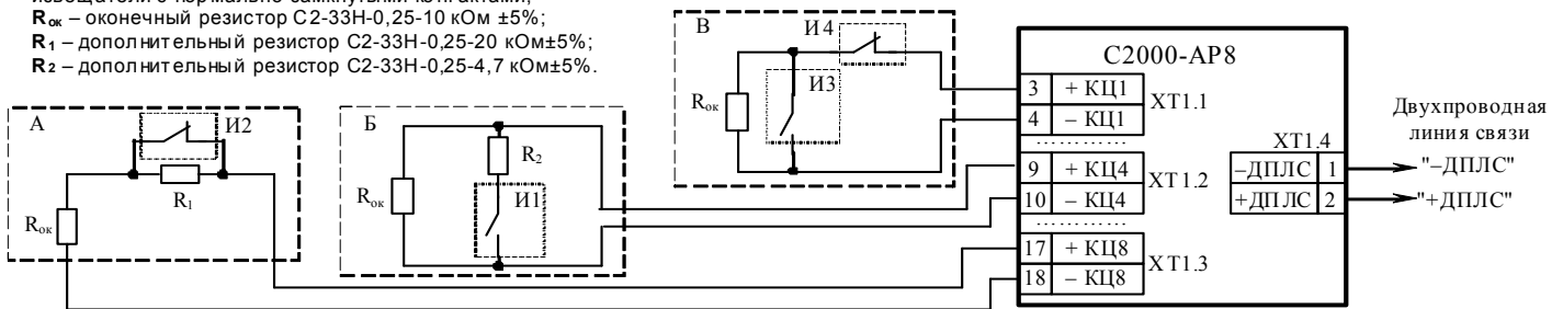
Рисунок 1 Схема соединений
