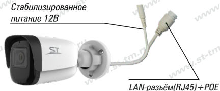
Рис.1 Схема подключения видеокмеры
