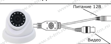
Рис.1 Схема подключения
