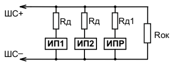
Пожарный ШС R d = 2 кОм ± 5%, 0,25 Вт – для ИП 212-41М, ИП 212-45, ИП 212-87; R d1 = 510 Ом ± 5%, 0,25 Вт – для ИПР 513-10; R ок = 4,7 кОм ± 5%, 0,25 Вт.
