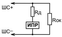
Локальный ШС R d = 510 Ом ± 5%, 0,25 Вт – для ИПР 513-10; R ок = 4,7 кОм ± 5%, 0,25 Вт.
