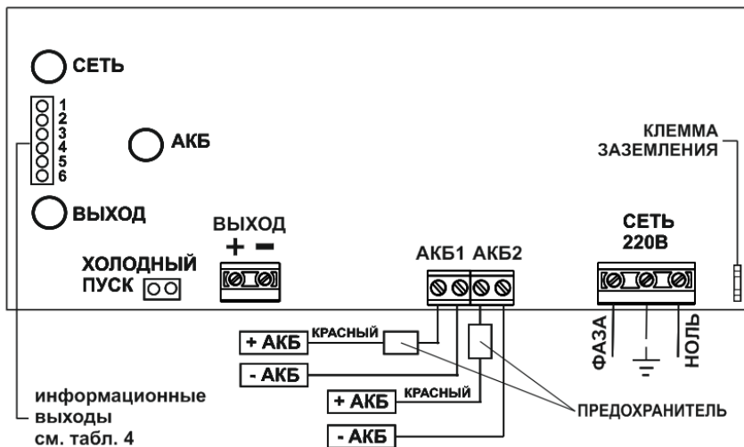
Рисунок 1. Вид источника с открытой крышкой (схема подключения)
