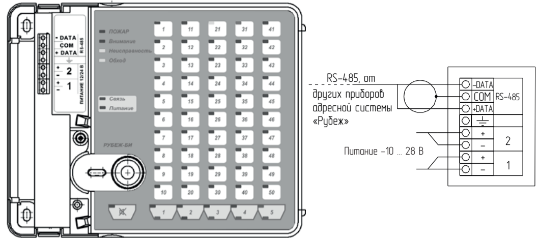
Рисунок 1 - Внешний вид и схема подключения прибора
