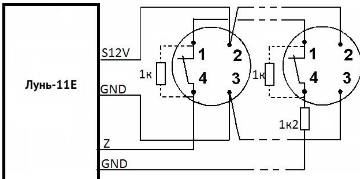
Рисунок 3. Схема подключения пожарных извещателей по четырехпроводной схеме
