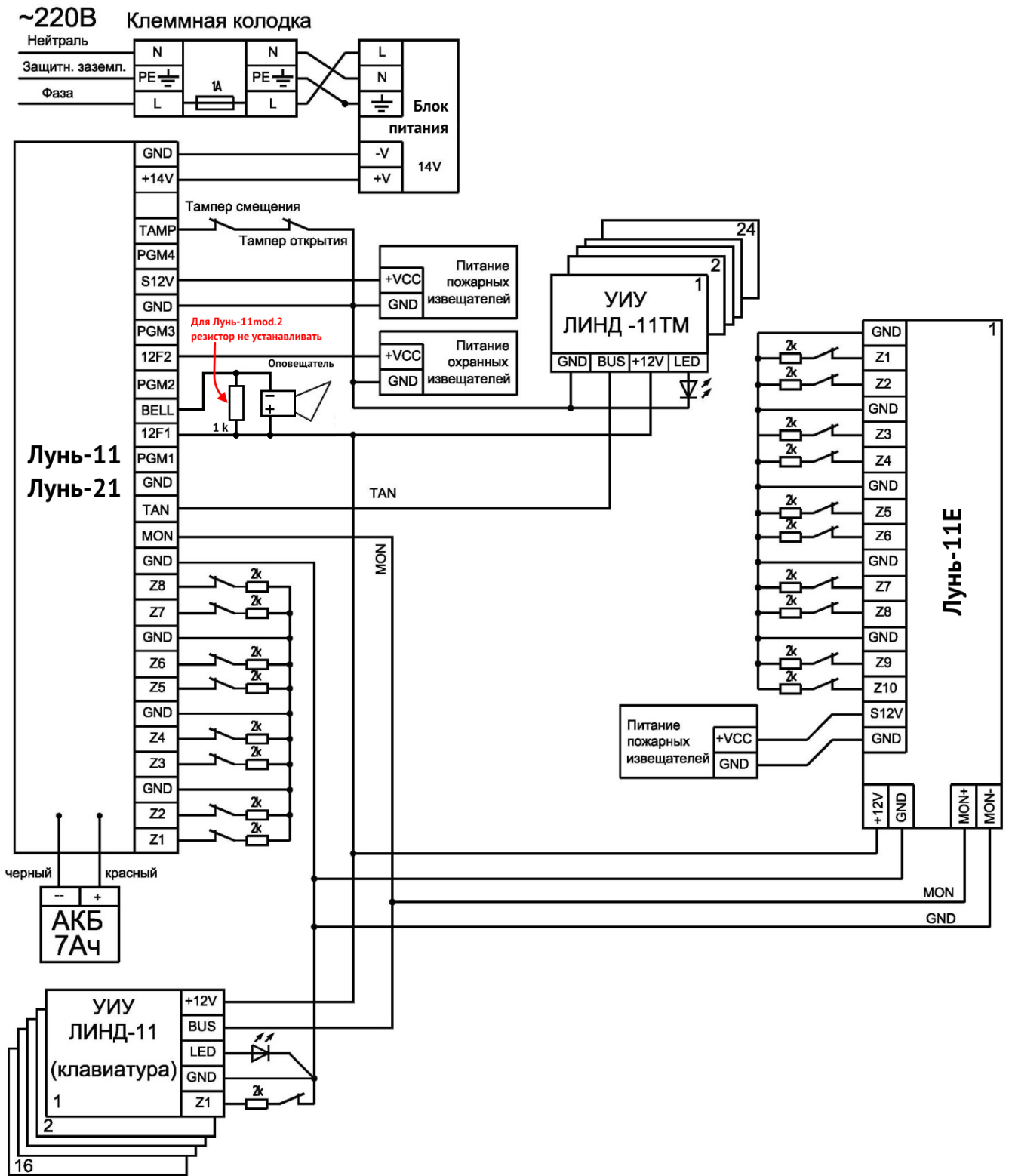
Рисунок 2. Схема подключения МР «Лунь-11Е»
