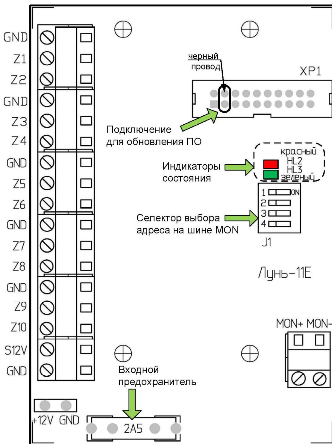
Рисунок 1. Внешний вид платы «Лунь-11Е»
