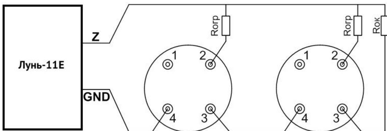
Рисунок 4. Схема подключения извещателей в пожарный шлейф по двухпроводной схеме
